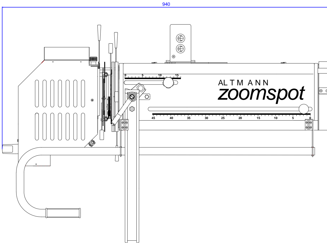
HMI-Zoom-Verfolgerscheinwerfer AZU 109 DMS Verdunklerblende (Dimmer) mit motorischem Antrieb und DMX-Ansteuerung Bei Bedarf: Zeichnung im DXF-Format bitte anfordern
